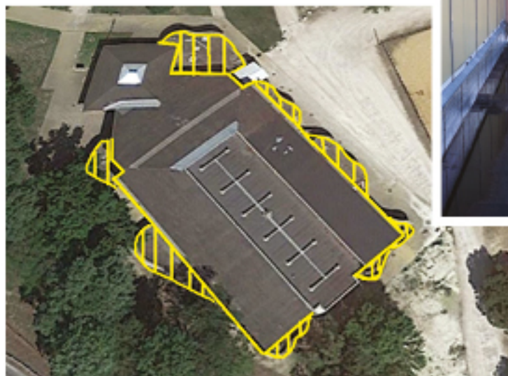
Réfection des toitures terrasses inaccessibles gravillonnées.
